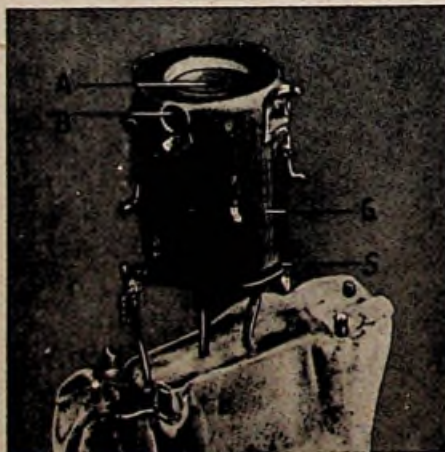
Abb. 5: Aufnahme des Wehneltzylinders der Elektronenstrahlröhre DG 9-3, G Wehneltzylinder, A Ausritzsöffnung für die Elektronen, B Beobachtungsöffnung zur Montage des Systems, S Abschirmung gegen Streu-Elektronen
