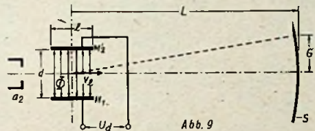
Abb. 9: Elektrodensystem zur elektrostatischen Strahlableitung. a_2 Anode, M_1 , M_2 Ablenkplatten, S Leuchtschirm.
