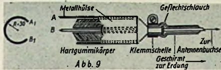
Abb. 9. Schnitt durch eine Tastenleiste zum Aufsuchen von Gehäuseundichtigkeiten bei Höchsthochfrequenzen. Ausführung B zum direkten Aufsetzen, wenn spannungsfreie Gehäuse vorliegen, anderenfalls ersetzt man zweckmäßig die Spitzen durch eine Drahtschleife Al-BI- (Fig. A)
