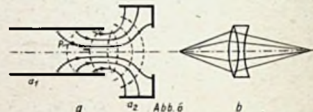
Abb. 6: Elektronenoptik — Lichtoptik, a) Spannungsverhältnisse zwischen Anode und Hilfsanode und ihr Einfluß auf den Elektronenstrahl; b) als Vergleich zu a) Gang der Lichtstrahlen in einer Glasoptik Zeichnungen: Trester
