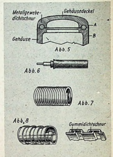
Abb. 5. Schnitt durch ein Apparategehäuse bei extremen Ansprüchen, für geringere Anforderungen genügt ein sauberer blanker Deckeinpaß. Abb. 6. Leitung mit Doppelgeflechtschlauch geschirmt. Abb. 7 (Richtig). Tombakwellenschlauch mit gelötetem Falz, Abb. 8 (Falsch) Gewöhnlicher Spiralschlauch
