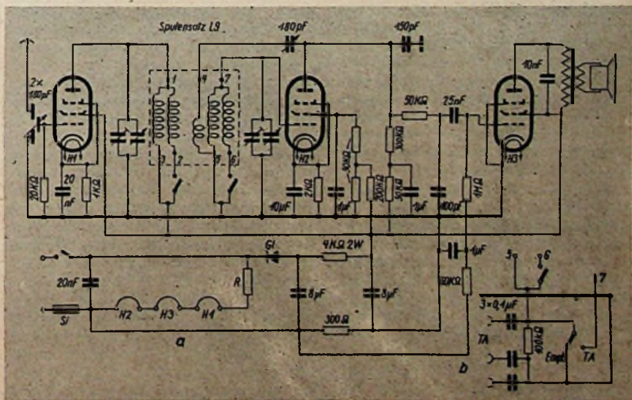
Abb. 3 a) Vollständiges Schaltbild, b) Umschaltung für Schallplattenanschluß
